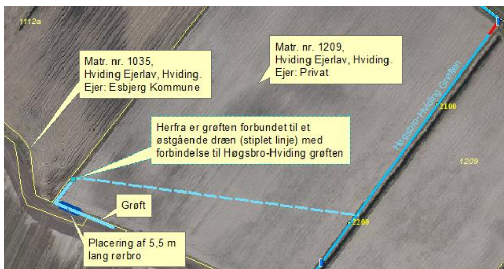
Figur 1. Placering af privat grøft og dræn med afløb til det offentlige vandløb Høgsbro-Hviding Grøften. Rørbroen ønskes placeret øst for grøftens 90 graders sving.
